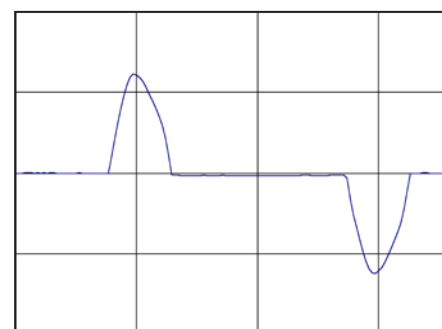
Figura 5. Corriente demandada por una carga electrónica
